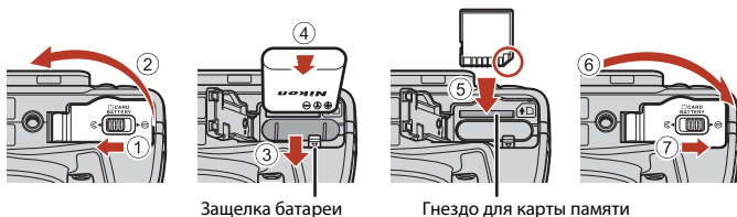
Защелка батареи
